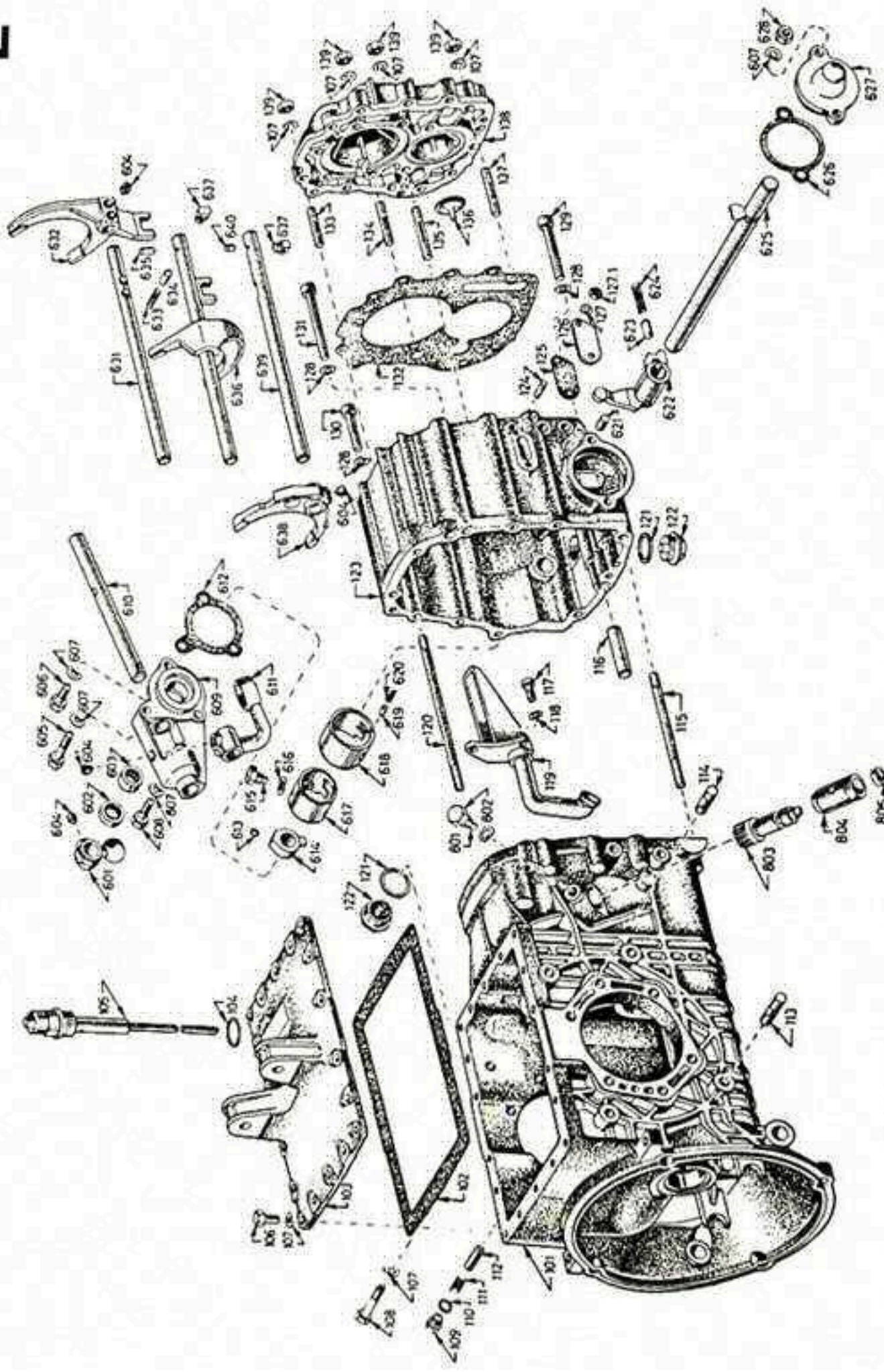
ZF Synchroma Gearbox 5 DS - 25
